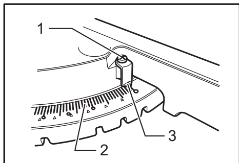
► 1. Tornillo 2. Escala de inglete 3. Puntero
