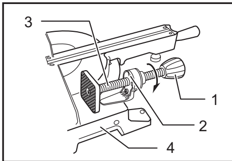
► 1. Bouton de l'étau 2. Partie saillante 3. Arbre de l'étau 4. Base
